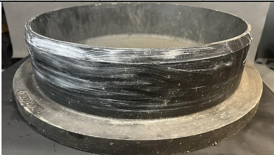
Rys.7 - Aplikacja smaru poślizgowego na zatyczce w celu poprawnej instalacji oraz zabezpieczeniu przed wywijaniem uszkodzeniem gumowej uszczelki - T4/600/Z.
