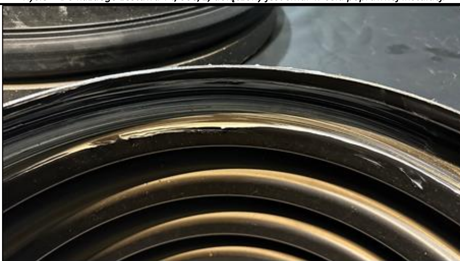
Rys.4 – Aplikacja smaru w celu instalacji uszczelki w najwyższym, wewnętrznym zagłębieniu rury korugowanej.
