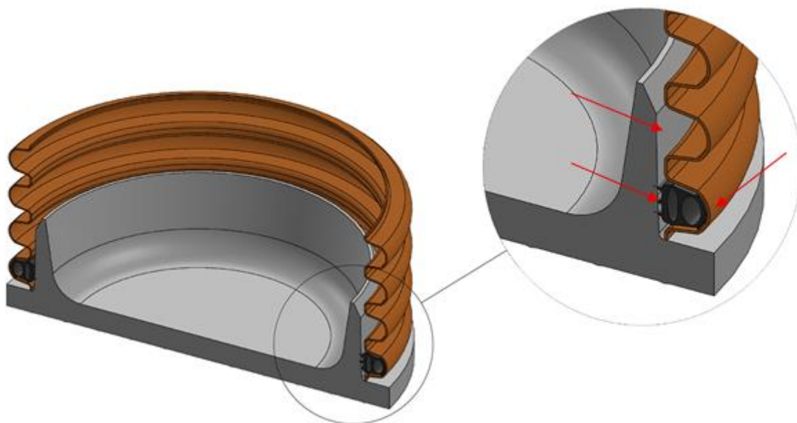
Rys.1 - Miejsce aplikacji smaru poślizgowego przy zatyczce T4/600/Z, systemu TVRT.
