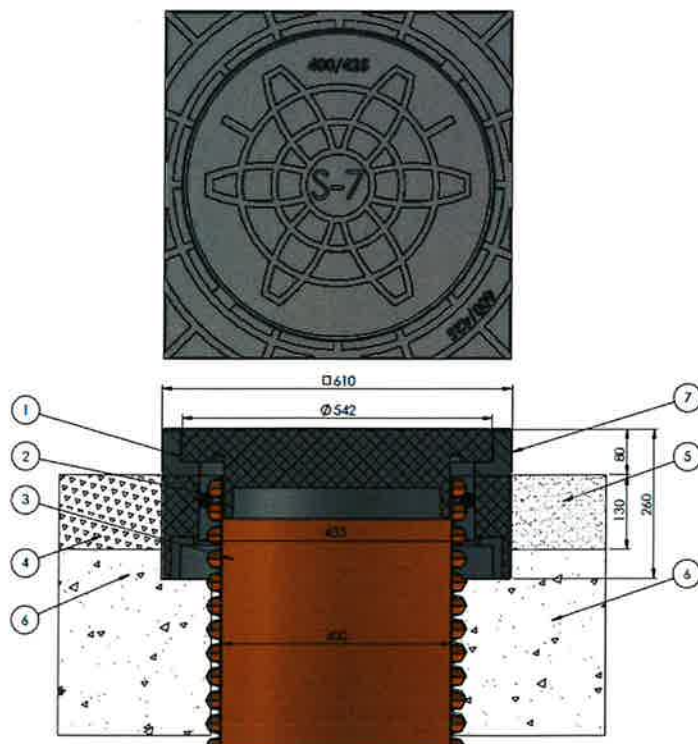
Rysunek Z-9 .Schemat posadowienia zwieńczenia zabezpieczającego T5/400/425/BB/UC. Elementy konstrukcji: 1) zwieńczenie T5/400/425/BB/UC osadzone na zagęszczonym gruncie wokół rury wznoszącej; 2) uszczelka między rurą trzonową a zwieńczeniem; 3) rura trzonowa SN4 DN/ID 400; 4) np. kruszywo kolejowe 5) np. grunt rodzimy, 6) zagęszczona obsypka piaskowa 93÷95% w skali Proctora, 7) Uwaga. zwieńczenie wyniesione 80 mm nad poziom terenu
