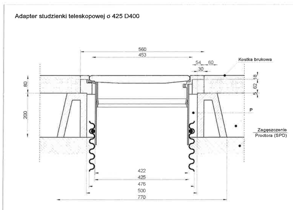
Rysunek Z-7 - Schemat posadowienia adaptera (typu 3) pod właz teleskopowy 425 TX425, wspartego na stożku odciażającym (typu 2) T3/425.
